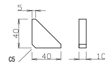
溶接補強リブ （配管接続部×8）
