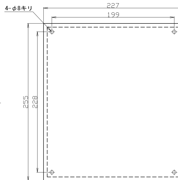
蓋寸法図
