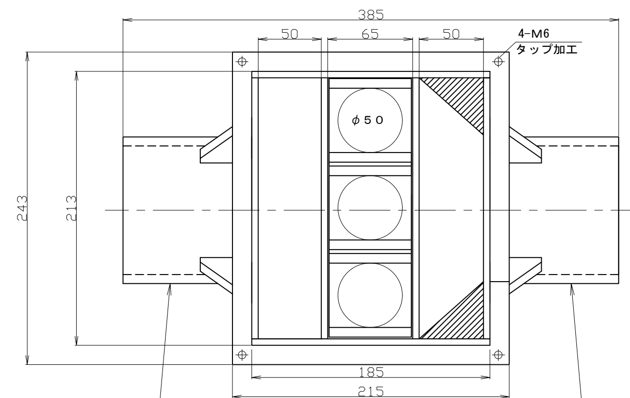
平面図（蓋ナシ）
