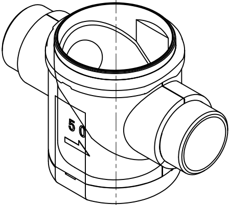
(2) 本体
