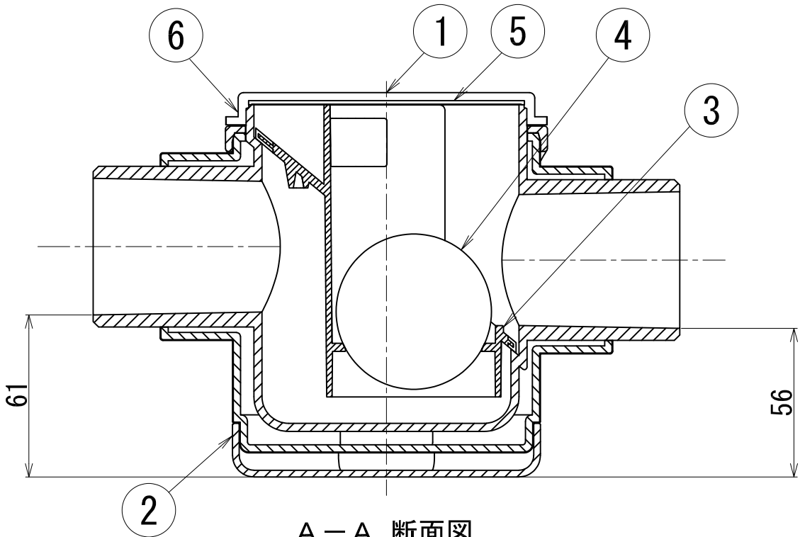
A-A 断面図
