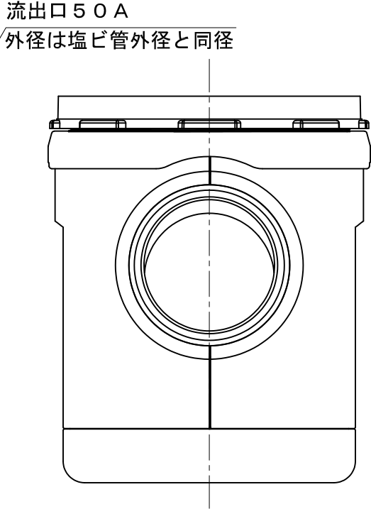
(2) 本体
