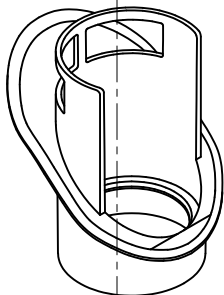
(4) 内部部品
