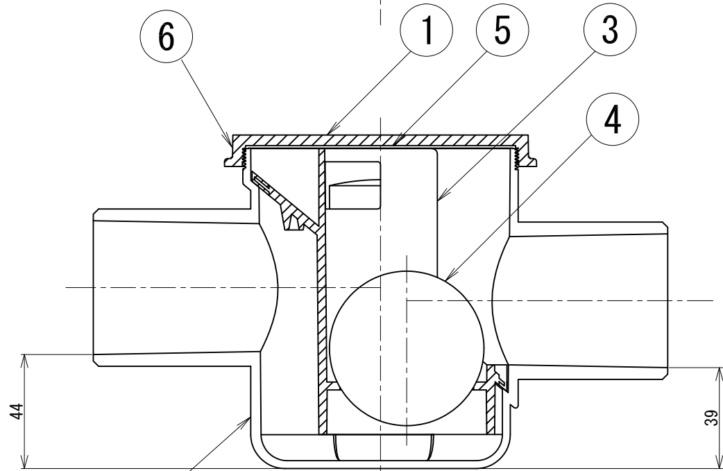
A-A 断面図
